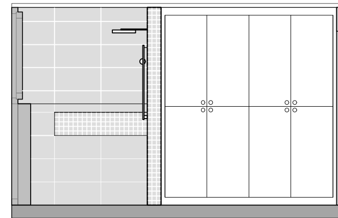
Ansicht Wand dusche
